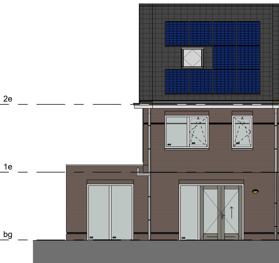
Achtergevel
